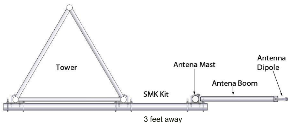
SMK-125-A3
