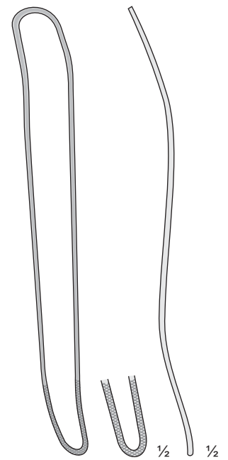
FRENZEL OM-19 165 mm
