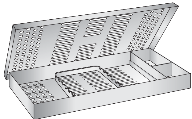
BS-42 285 x 190 x 25 mm Con griglia e scomparti
