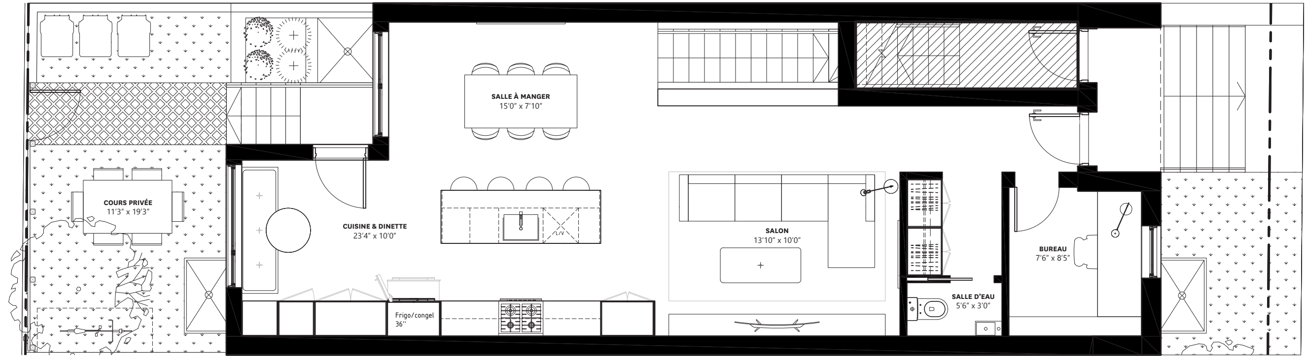
REZ-DE-CHAUSSÉE
