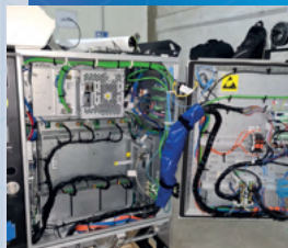
Gabinete Eléctrico
