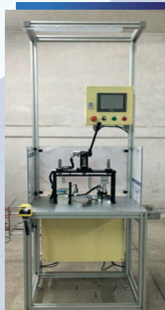
Estación para prensado manual de levas. DENSO
