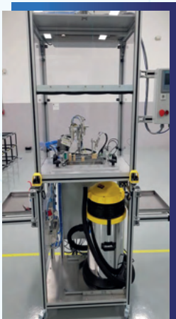
Estación de limpieza con aire ionizado. F&P
