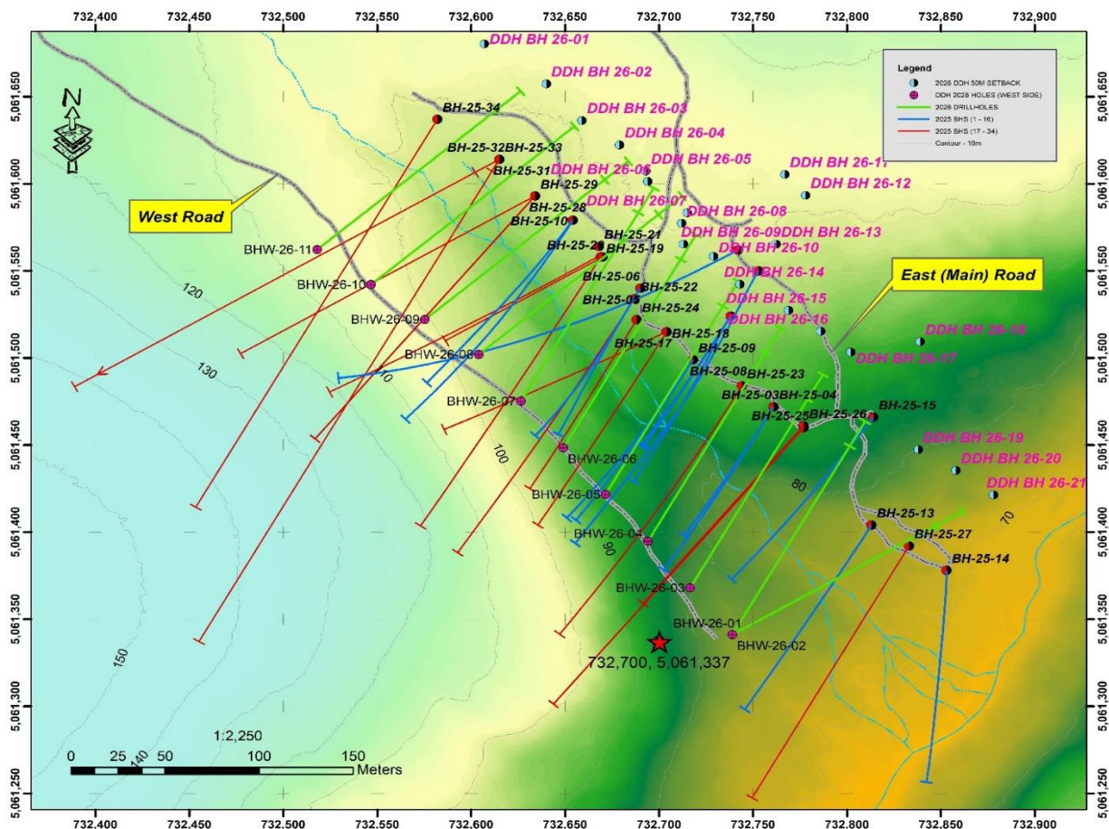
Abbildung 1: Detaillierter Bohrplan für Definitionsbohrungen
