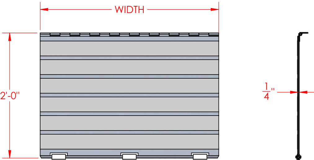
APRON PLATE
