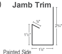
⑰ Jamb Trim
