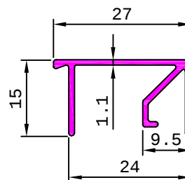
19385 0.216 kg/m
