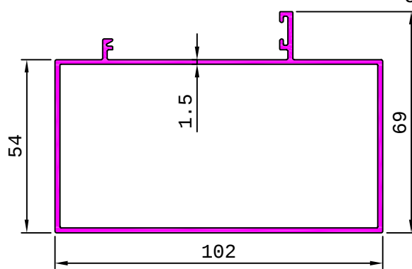
S5485 1.367 kg/m
