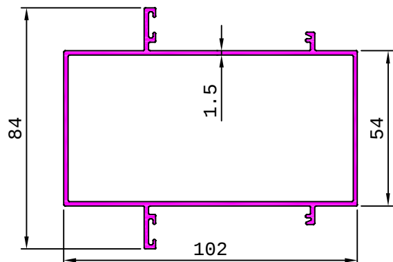
S5486 1.495 kg/m
