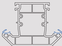
702504 95mm T Transom
