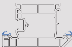
705511 110mm Door Sash Open Out
