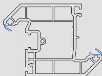
705515 95mm Z Transom / Slim Door Sash
