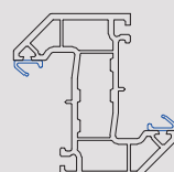
702506 70mm Z Transom
