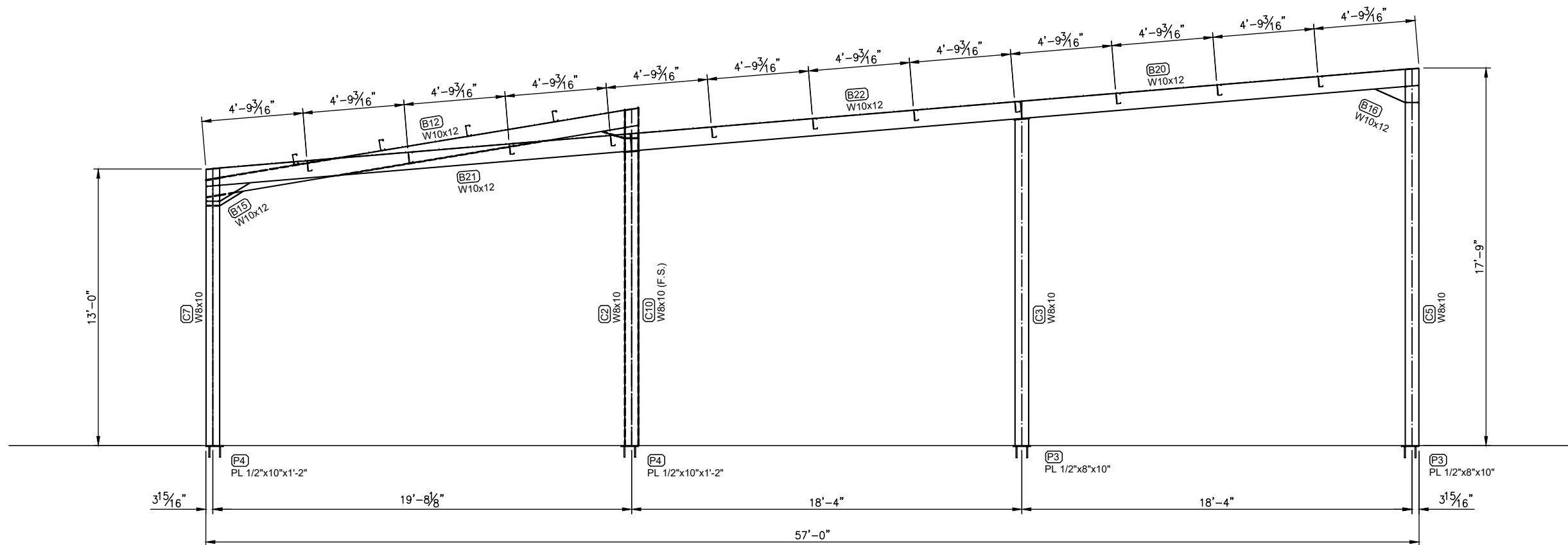
SECTION 2 SCALE: 3/8"=1'-0" BA-E3
