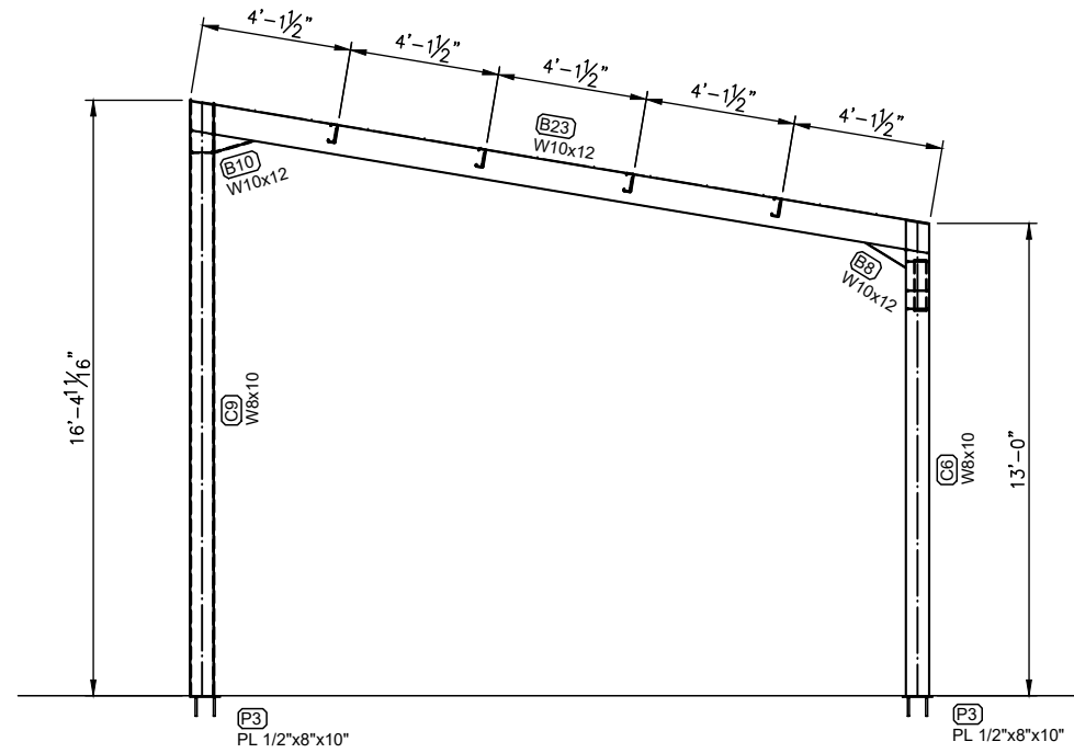
SECTION 4 SCALE: 3/8"=1'-0"
