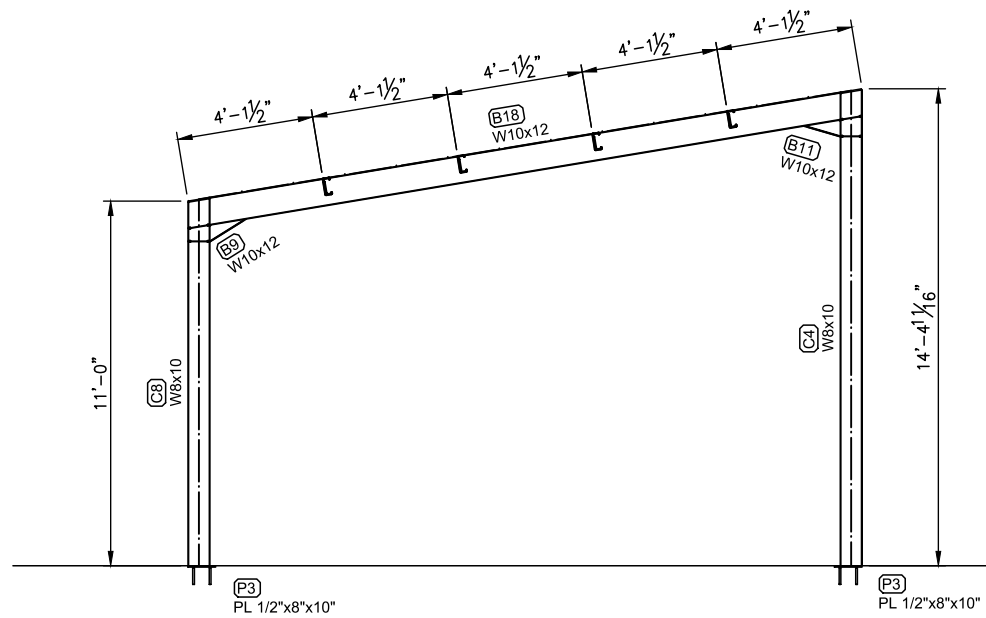
SECTION 3 SCALE: 3/8"=1'-0"
