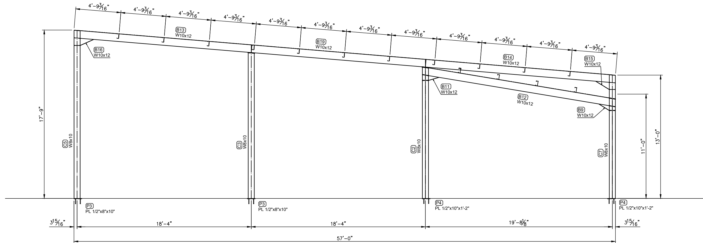
SECTION 1 SCALE: 3/8"=1'-0" BA-E3
