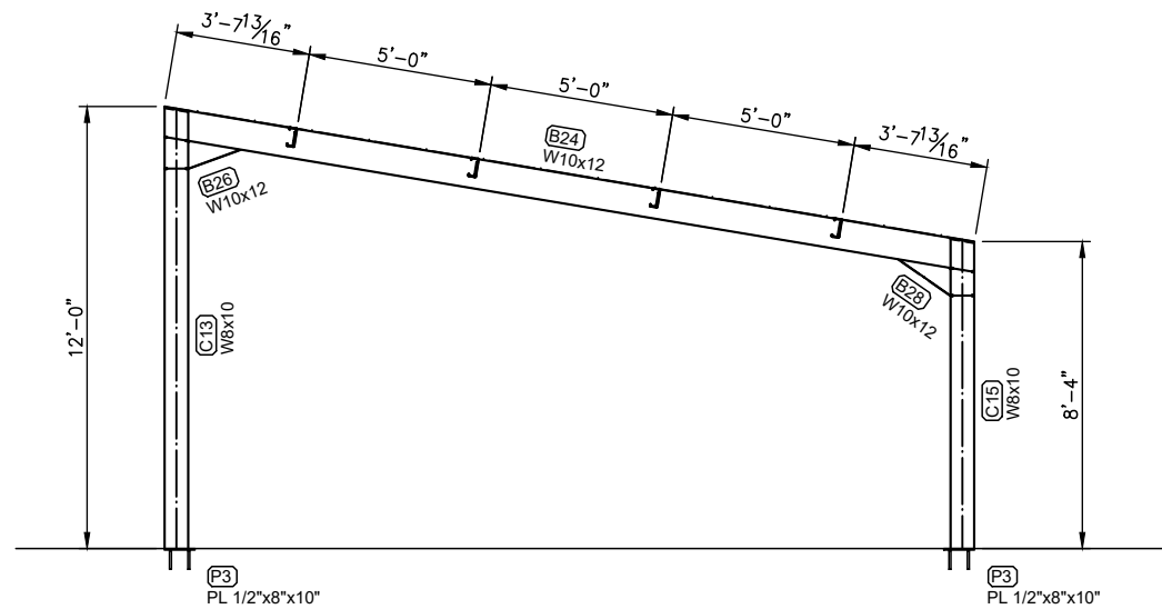
SECTION 5 SCALE: 3/8"=1'-0"
