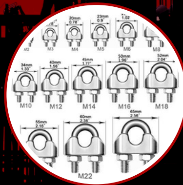
G.I & M.S U Clamps
