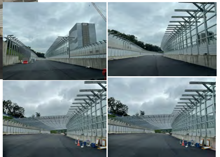
◀ 방음터널
