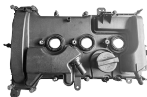
Tapa de Punterías, PCV y Tapon Incluido Ford Figo 1.5L 3 Cil 19-22
