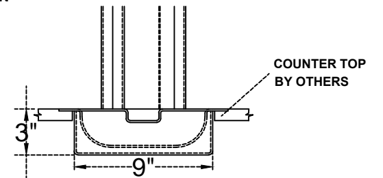
OPTIONAL MORTISE SILL SECTION
