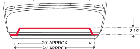
1930-1931 FORD FIREWALL 2 1/2" SET-BACK 301005 2 1/2" SET-BACK
