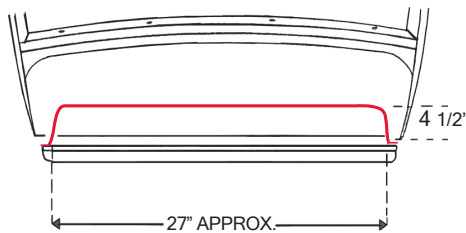
301000 1930-31 FORD FIREWALL (4 1/2" Set-Back)
