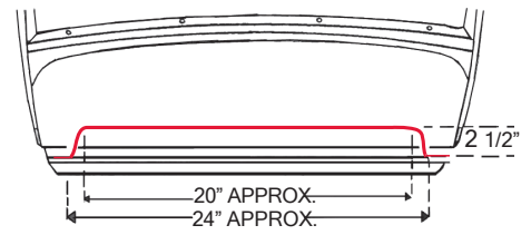
301005 1930-31 FORD FIREWALL (2 1/2" Set-Back)
