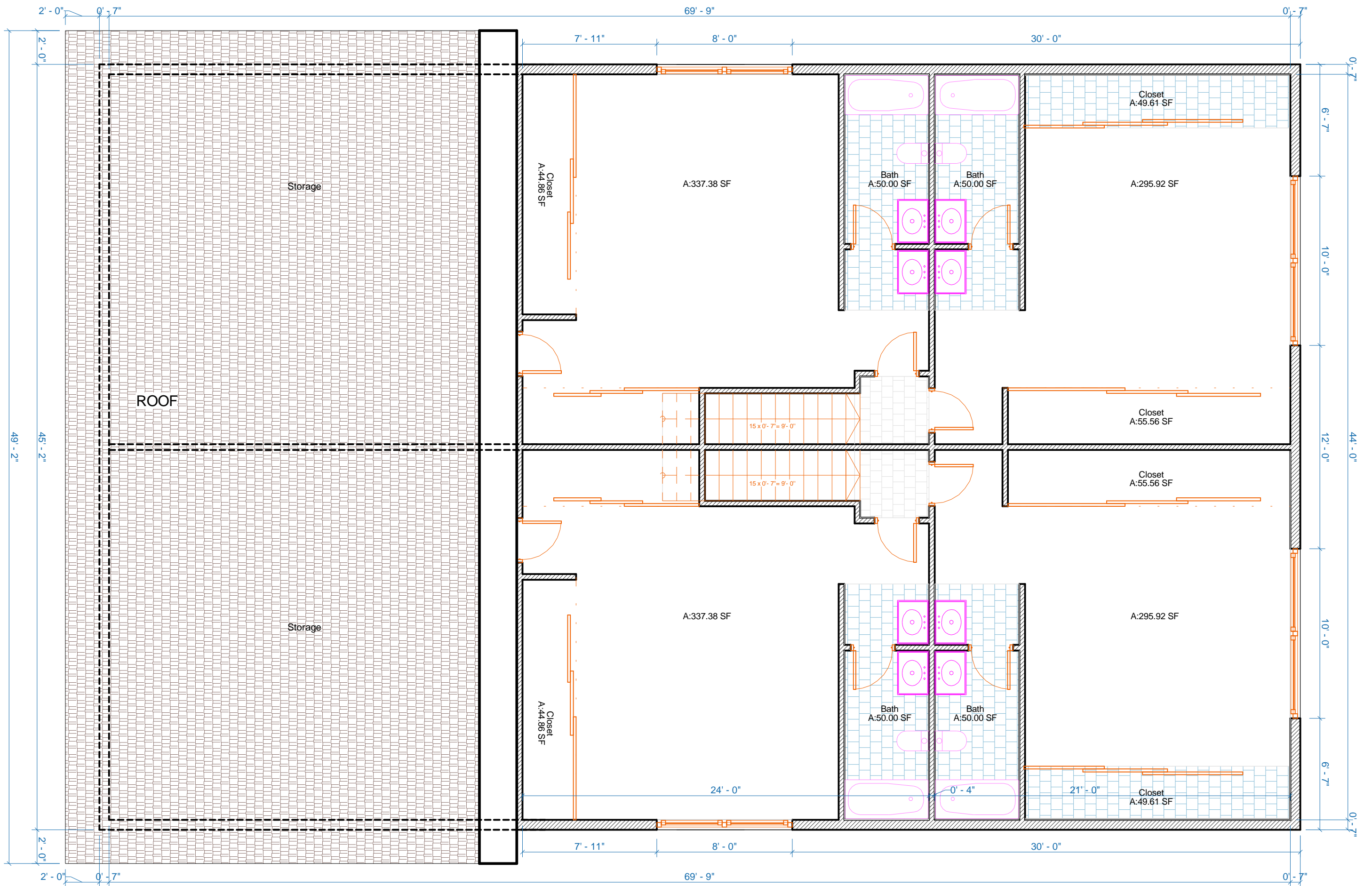
Level 3 Scale: 1' - 0"
