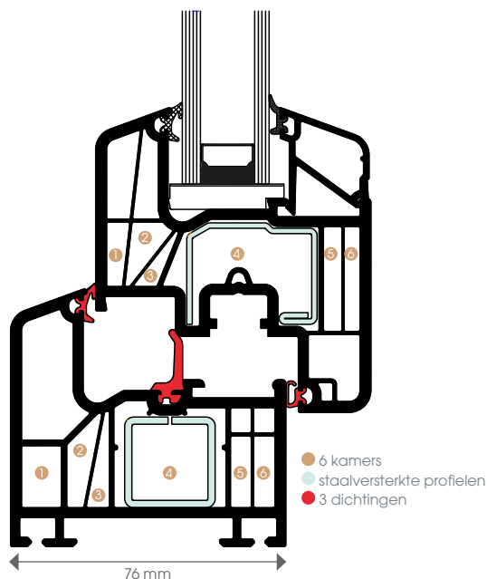
Fig. 1: staalversterkingen, 3 dichtingen en 6 kamers
