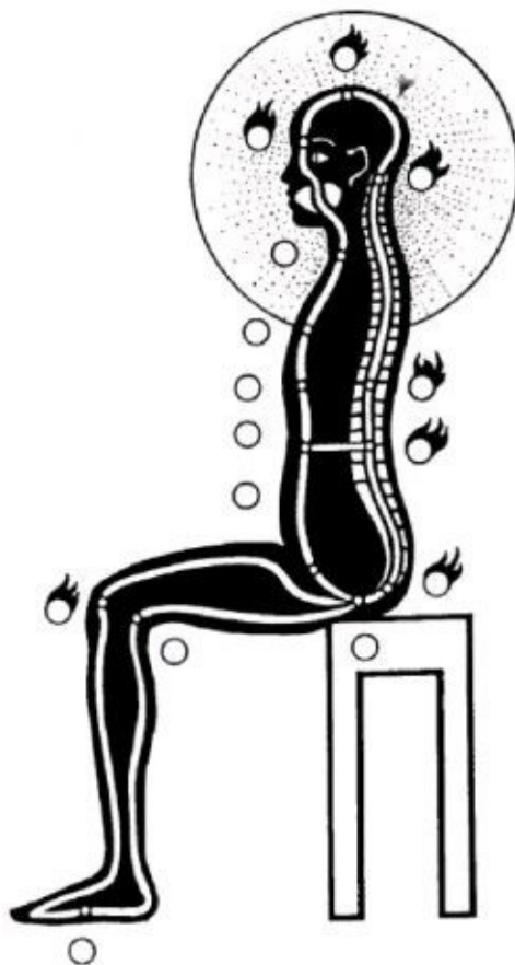
Fig. 32. — L'Orbite Microcosmique.
