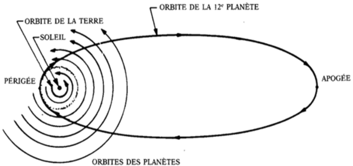
ORBITES DES PLANETES DU SYSTEME SOLAIRE
