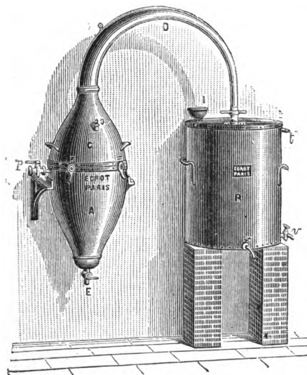
Fig. 43. — Œuf rectificateur perfectionné par M. Egot.
