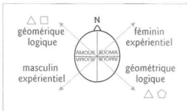
Illustration 4-3. Les régions qui se réfléchissent, en avant et en arrière.
