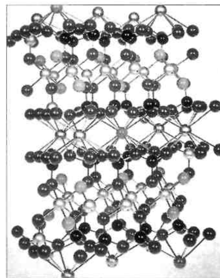
Illustration 6-33. Formation moléculaire compliquée.
