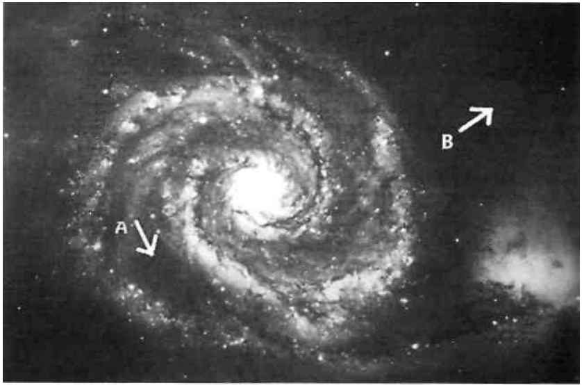
Illustration 2-35. Galaxie en spirale.
