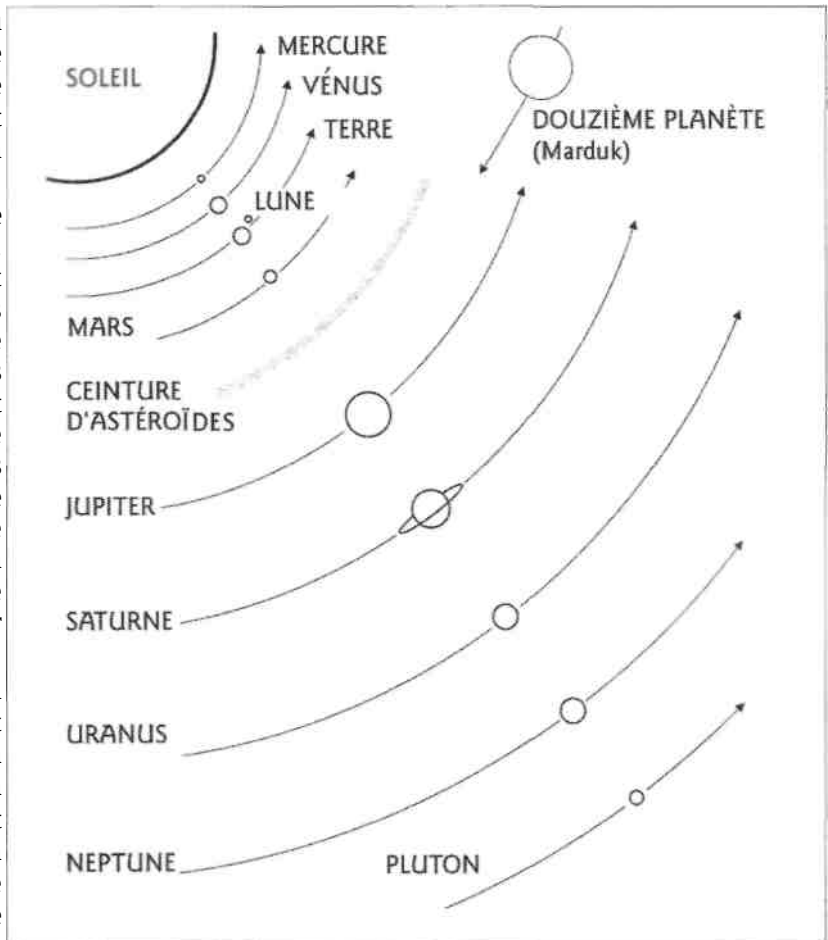
Illustration 3-8. Le système solaire, y compris Nibirou/Marduk et ce qui reste de Tiamat (la ceinture d'astéroïdes et la Terre).
