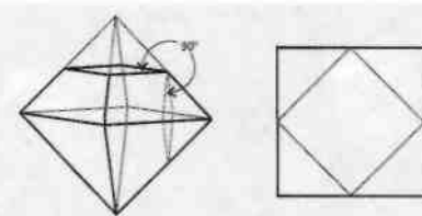
Illustration 6-40. Observation de la facette (à droite) créée en retranchant les six pointes d'un octaèdre. À gauche, nous présentons ce dernier avec une seule pointe tronquée, ainsi qu'une autre en pointillé à 90 degrés de la première.
