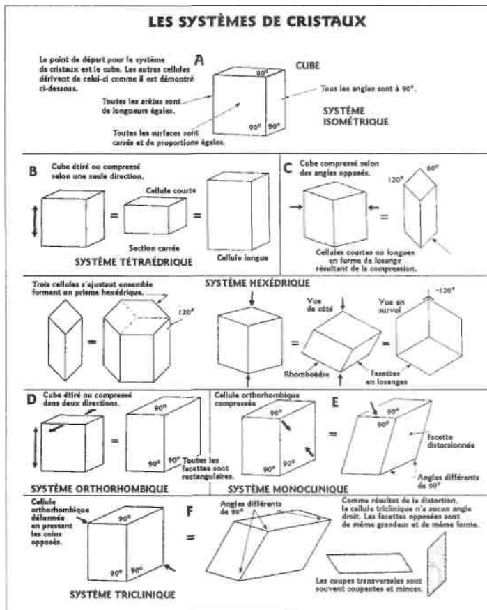
Illustration 6-34. Les systèmes de cristaux.
