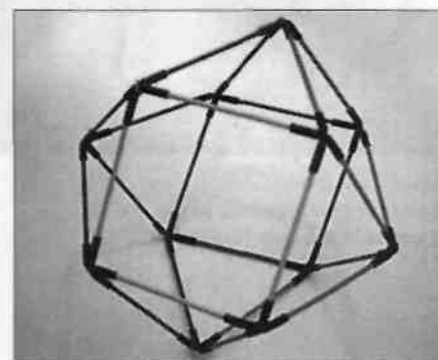
Illustration 6-42. Vecteur ou cube équilibre sous la forme d'un jouet qu'on appelle le Vector Flexor.
