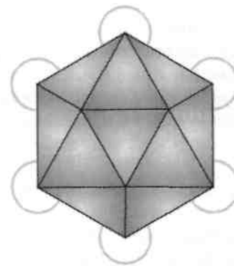
Illustration 6-19a. Le grand icosaèdre rendu plus visible.
