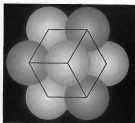
Illustration 6-8a. Cube formé des lignes qui passent par le centre de chaque sphère.
