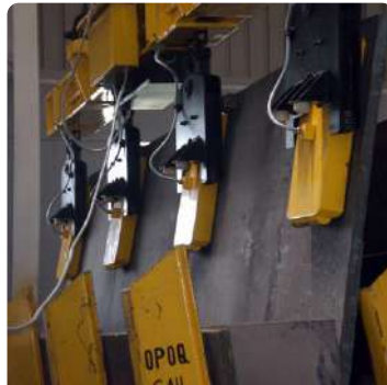
EM Horizontal/ Vertical Plate Handling
