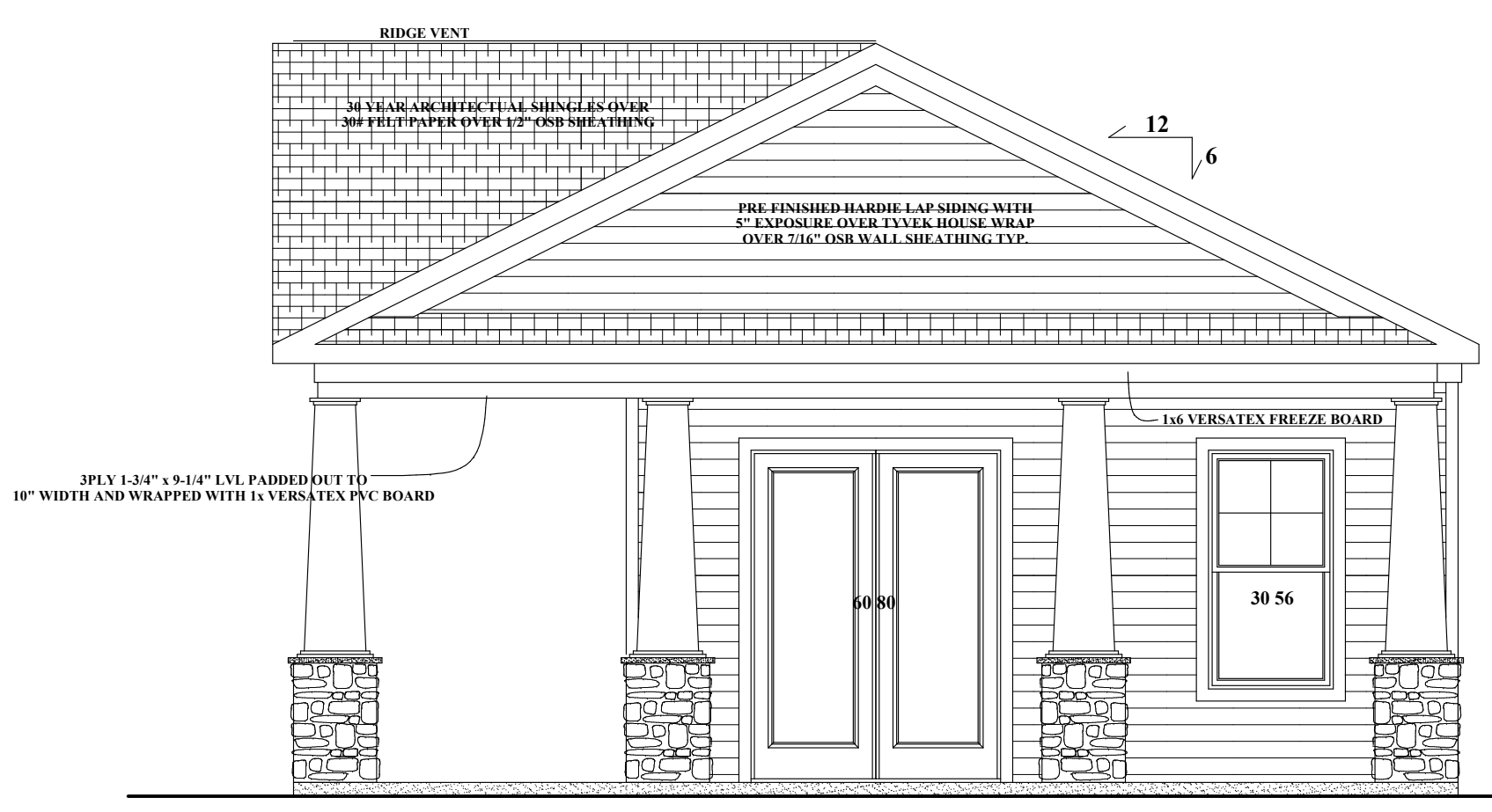
RIGHT ELEVATION
