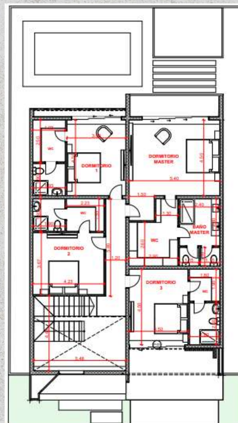
PLANTA ALTA
