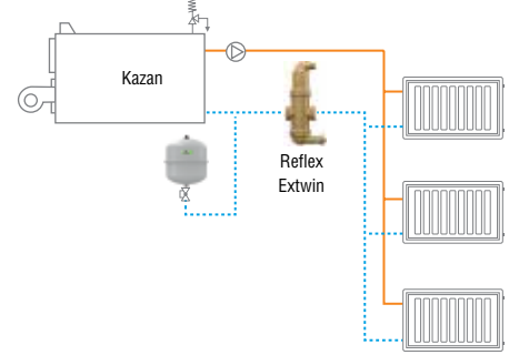
Extwin "pirinç" sistemi birleşik mikro kabarcık, tortu ve pislik ayırma şeması
