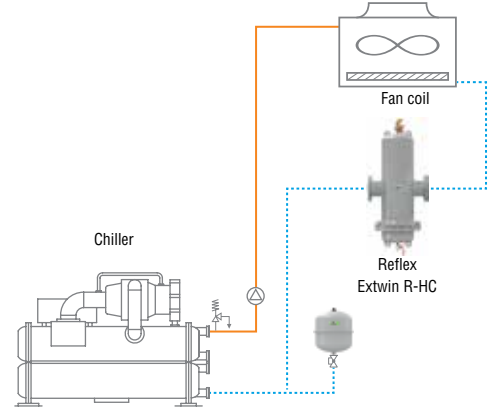
Extwin "Çelik" HiCap kontrol açıklıklı sistem birleşik mikro kabarcık, tortu ve pislik ayırma şeması
