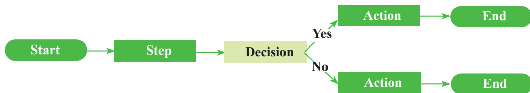
Fig. 5.22 : Flow Chart
