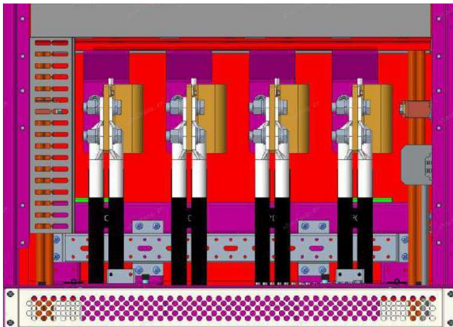
Figura 6.6.5 (1) Porta di interfaccia Schema del cavo DC sull'armadio integrato I modelli consigliati
