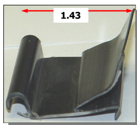
109-184 Screen clip-bottom
