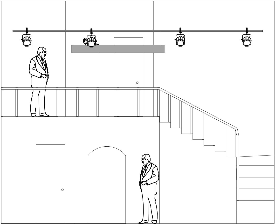
1 Elevation Scale: 1/4" = 1'-0"
