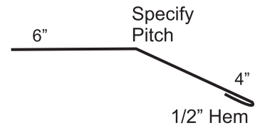
Gambrel
