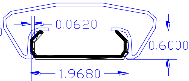
CLIP MOLDURA
