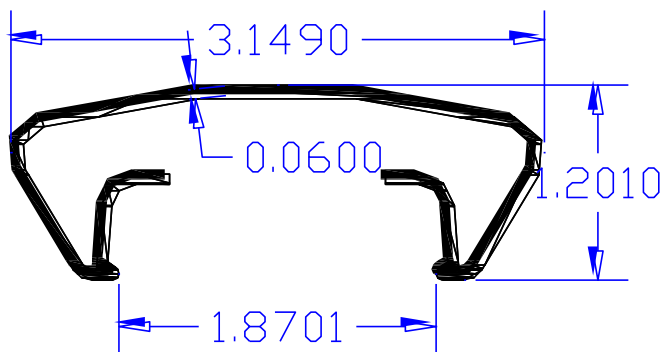
MOLDURA PASAMANOS
