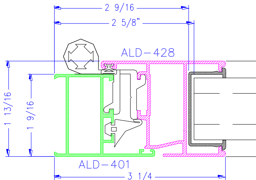
SECCION HORIZONTAL.
