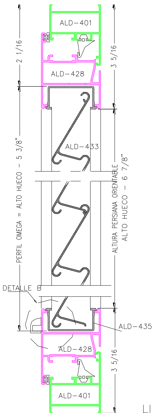
SECCION VERTICAL.
