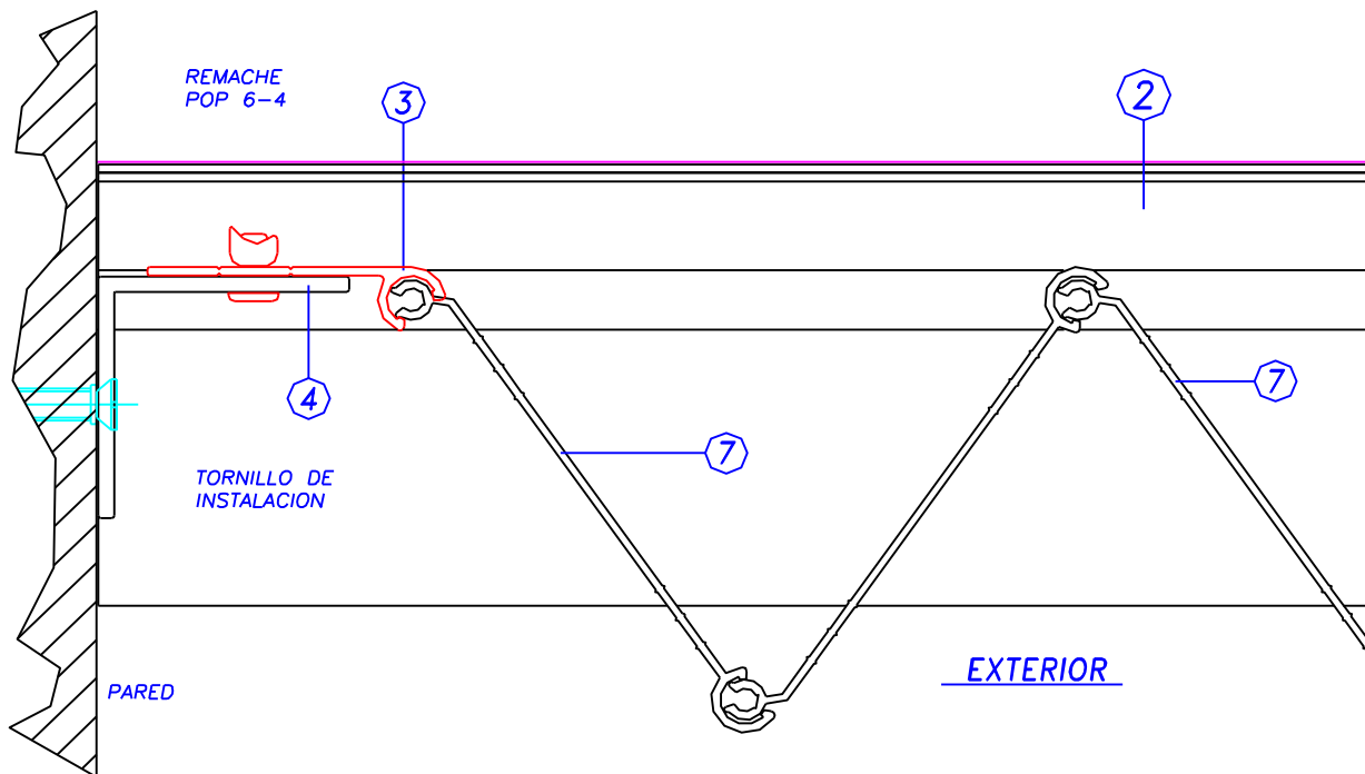
① CORTE HORIZONTAL DETALLE RTE LATERAL
