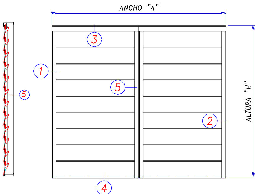
VENTANA DE CELOZIA VIDRIO
