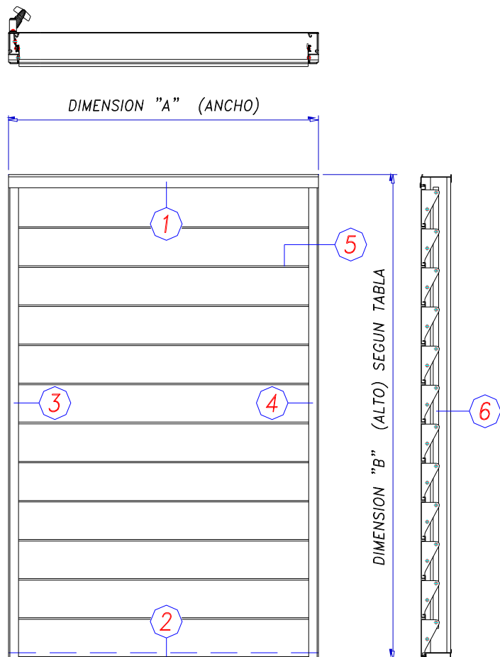
VENTANA DE CELOSLA
