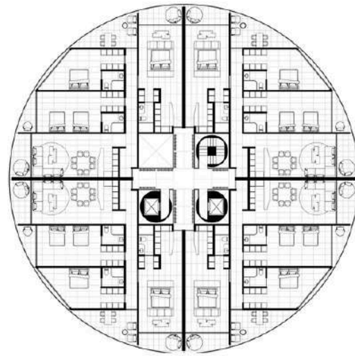
Las Palmas residencial Planta Tipo
