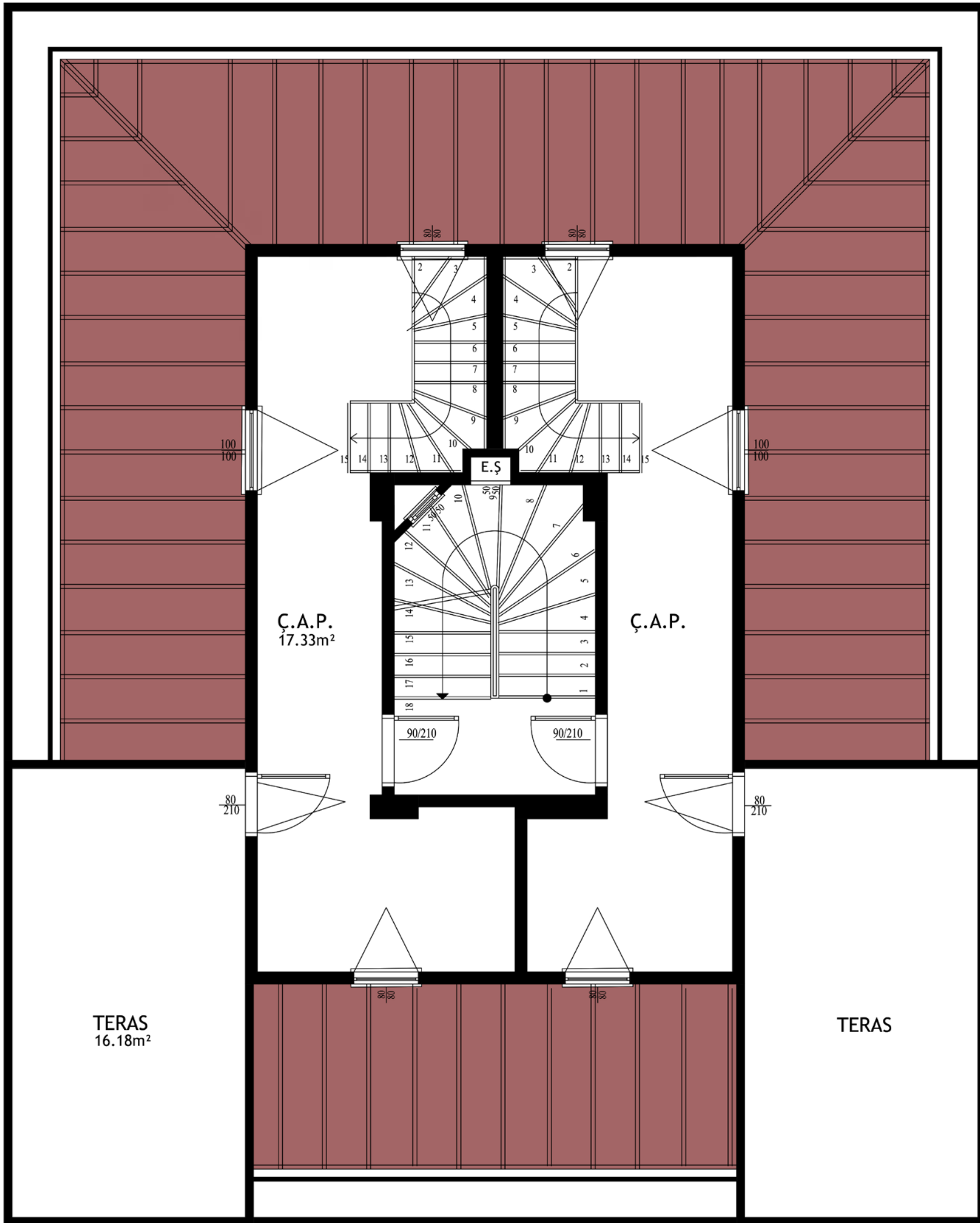
ÇATI KATI PLANI
