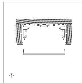
② 直接嵌入槽中 Insert directly into the slot
