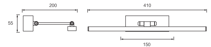
Dimension(mm)
