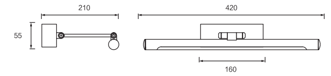
Dimension(mm)
