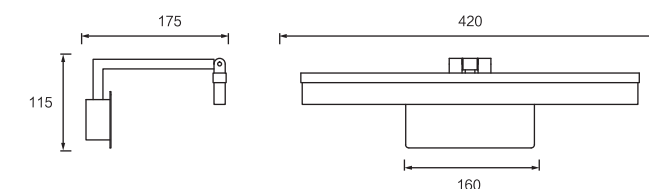
Dimension(mm)
