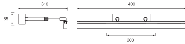
Dimension(mm)
