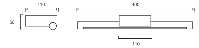
Dimension(mm)
