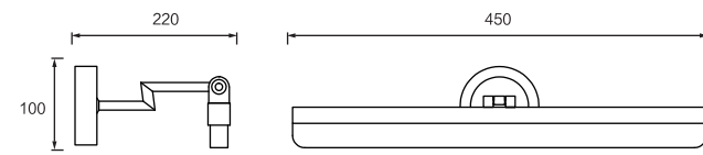
Dimension(mm)
