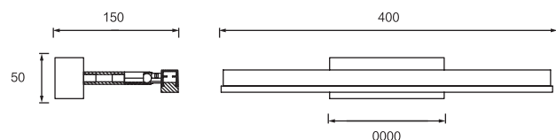
Dimension(mm)
