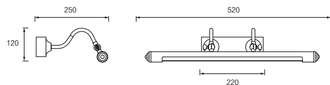
Dimension(mm)
