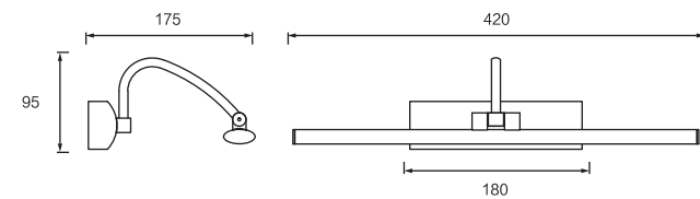
Dimension(mm)
