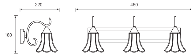
Dimension(mm)
