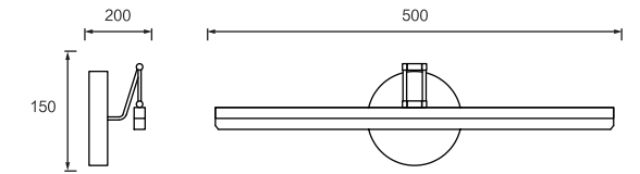
Dimension(mm)
