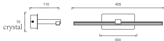
Dimension(mm)
