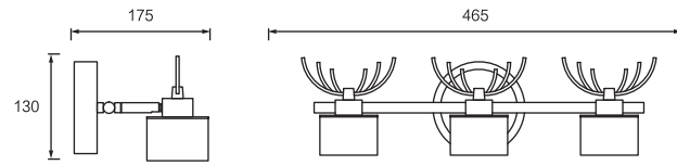
Dimension(mm)
