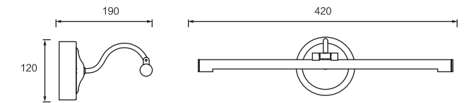
Dimension(mm)
