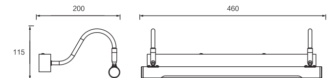
Dimension(mm)
