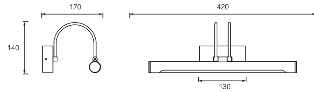
Dimension(mm)
