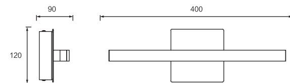
Dimension(mm)
