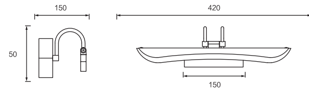
Dimension(mm)
