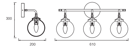
Dimension(mm)
