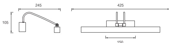
Dimension(mm)
