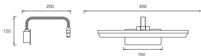
Dimension(mm)
