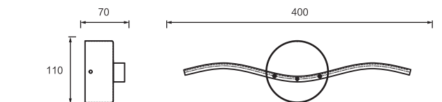
Dimension(mm)
