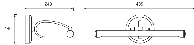
Dimension(mm)
