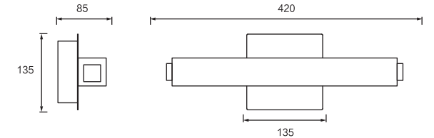
Dimension(mm)
