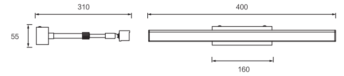
Dimension(mm)
