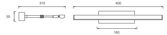
Dimension(mm)
