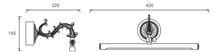
Dimension(mm)
