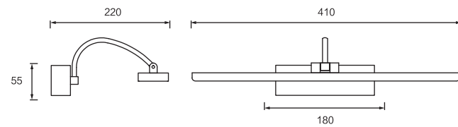
Dimension(mm)
