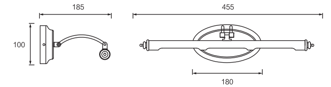
Dimension(mm)
