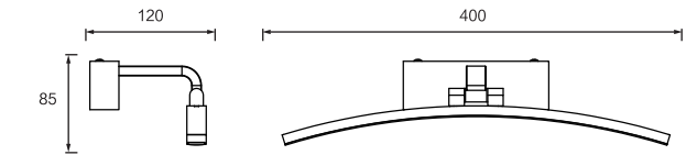
Dimension(mm)
