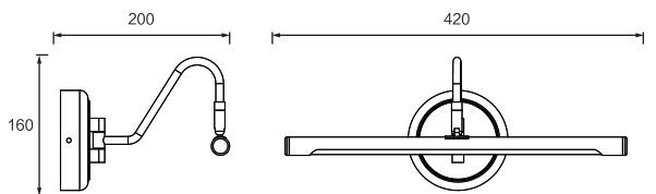
Dimension(mm)
