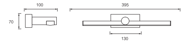
Dimension(mm)
