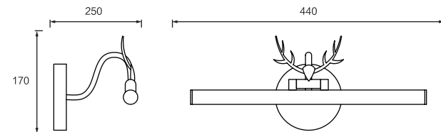
Dimension(mm)
