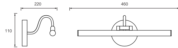
Dimension(mm)
