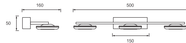
Dimension(mm)
