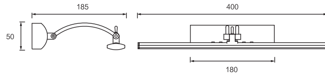
Dimension(mm)
