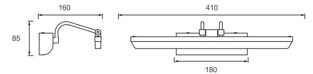
Dimension(mm)
