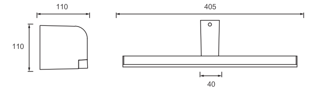
Dimension(mm)
