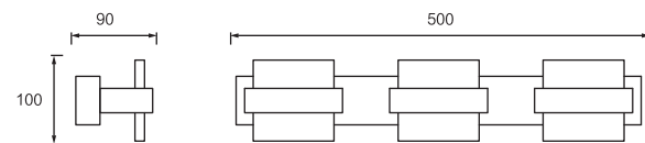
Dimension(mm)
