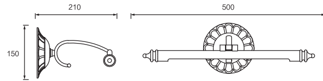
Dimension(mm)
