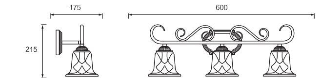
Dimension(mm)
