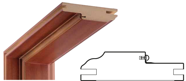
CERCO MOLDURADO REGULABLE CON BURLETE MOLDED ADJUSTABLE FENCE WITH WEATHERSTRIP CLÔTURE MOULÉE RÉGLABLE AVEC BANDE MÉTÉO
