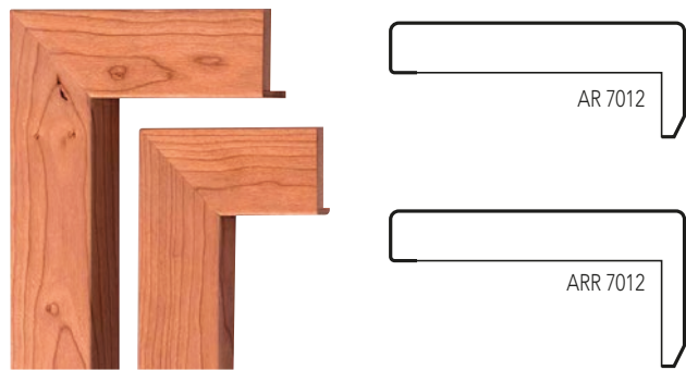
MOLDURA RECTA EXTENSIBLE STRAIGHT EXTENDABLE MOLDING MOULURE DROITE EXTENSIBLE
