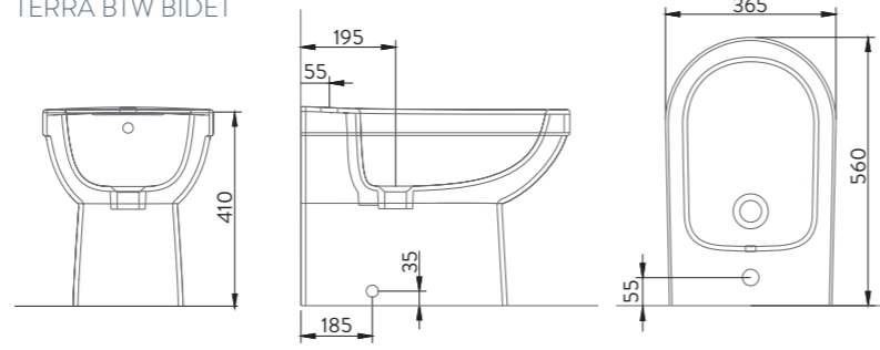
A017001H TERRA YERDEN BİDE TERRA BTW BIDET
