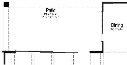
Opt. 16' Center Sliding Door
