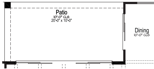
Opt. 15' Multi-Slide Door
