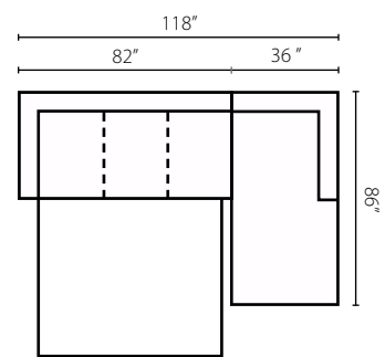
Configuration C E16L DQSL One Arm Queen Sleeper E16R CHASE One Arm Chaise
