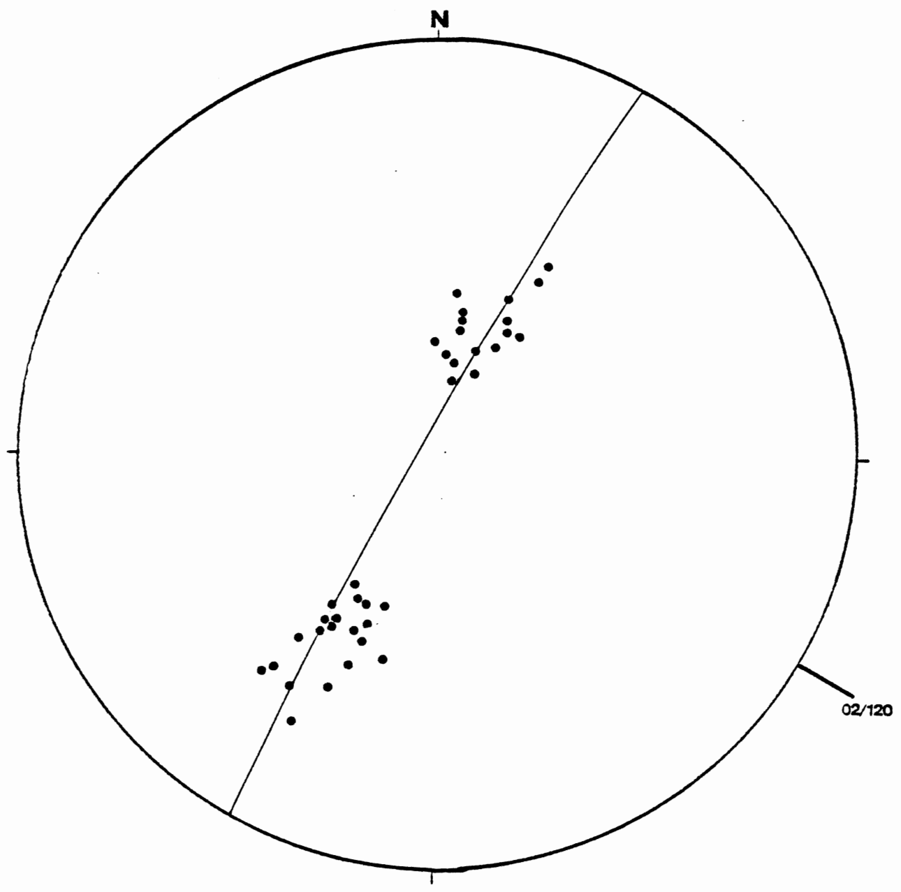
White Tail Anticline (WA)
