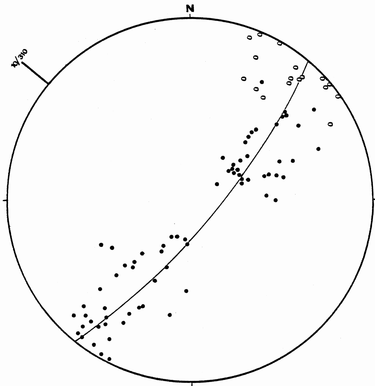
Kiowa Syncline (KS)
