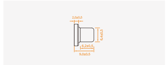
Integral end cap
