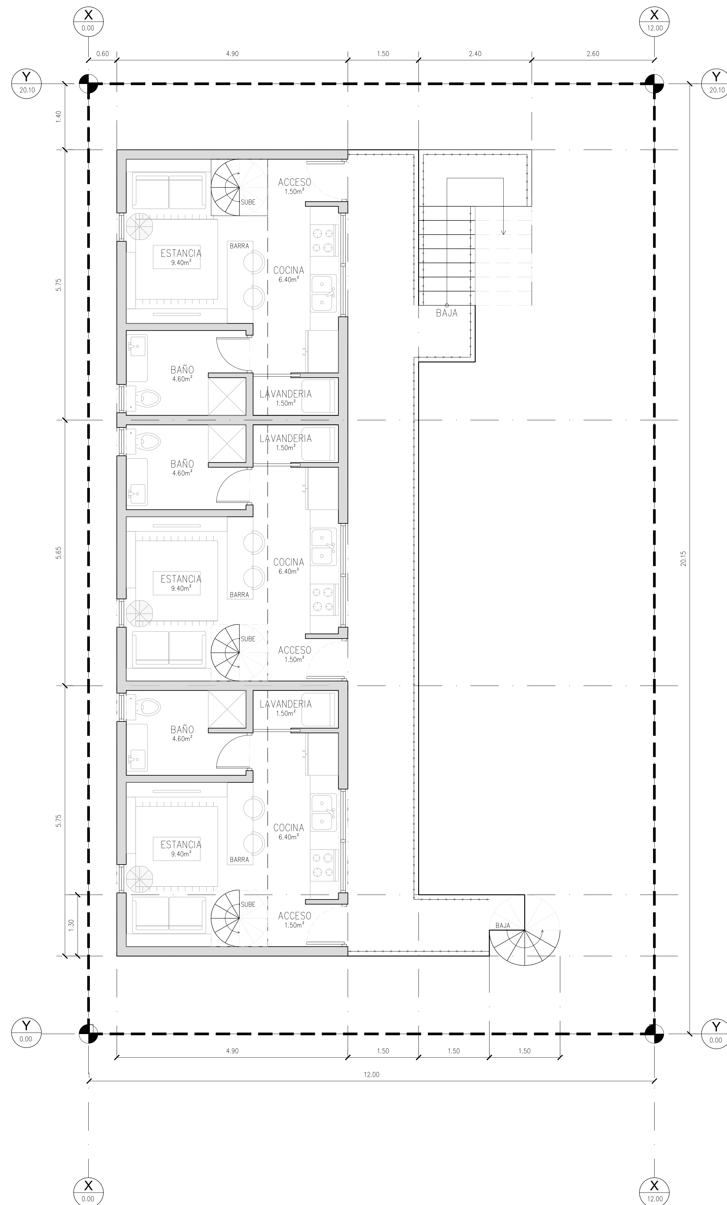
PLANTA ARQUITECTONICA - 2do NIVEL
