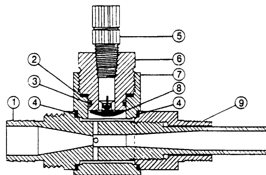
EJECTOR MODEL A-925S
