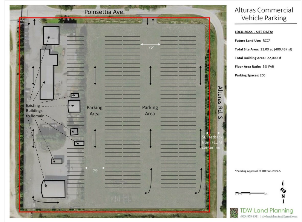
Site Plan 7621 bartow
