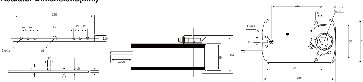
Actuator Dimensions(mm)
