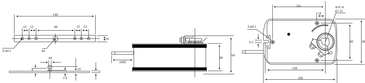
Actuator Dimensions(mm)
