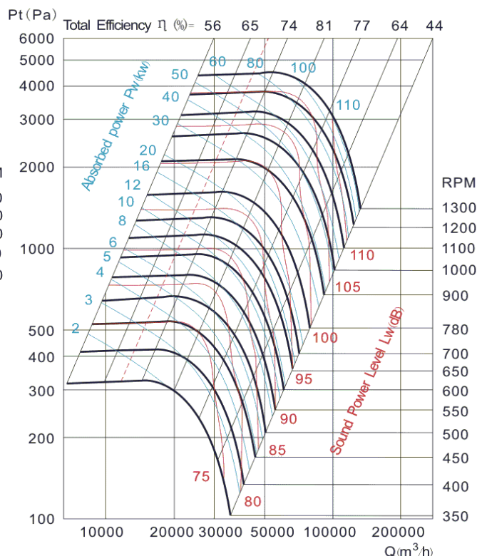
CBA-BA-1400BS-X-X-X
