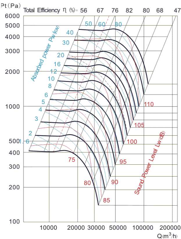
CBA-BS-800BD-X-X-X
