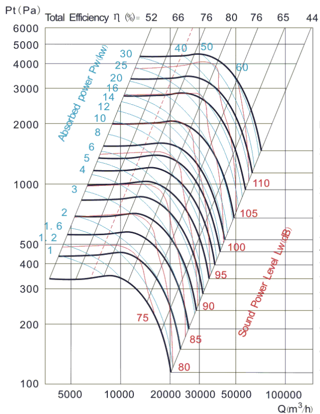
CBA-BS-630BD-X-X-X
