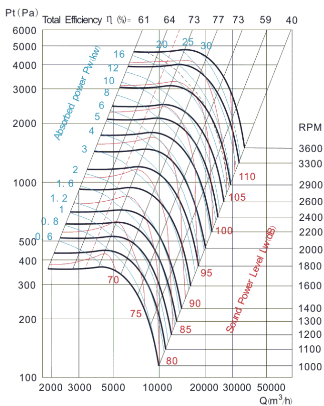
CBA-BS-450BD-X-X-X
