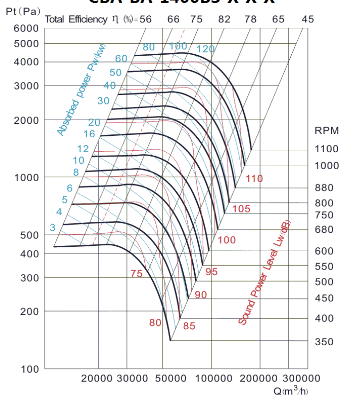
CBA-BA-1400BS-X-X-X
