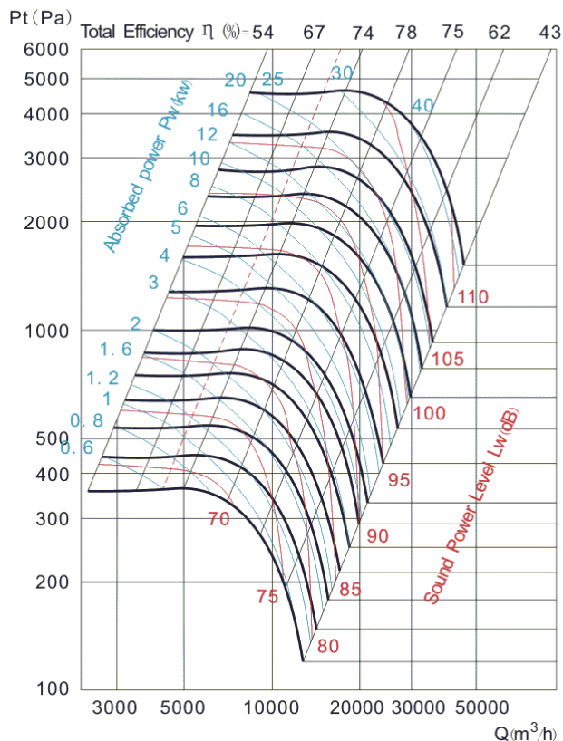
CBA-BS-630BD-X-X-X
