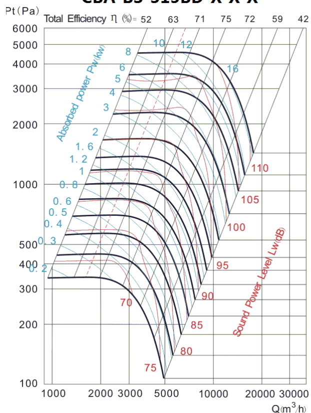
CBA-BS-315BD-X-X-X
