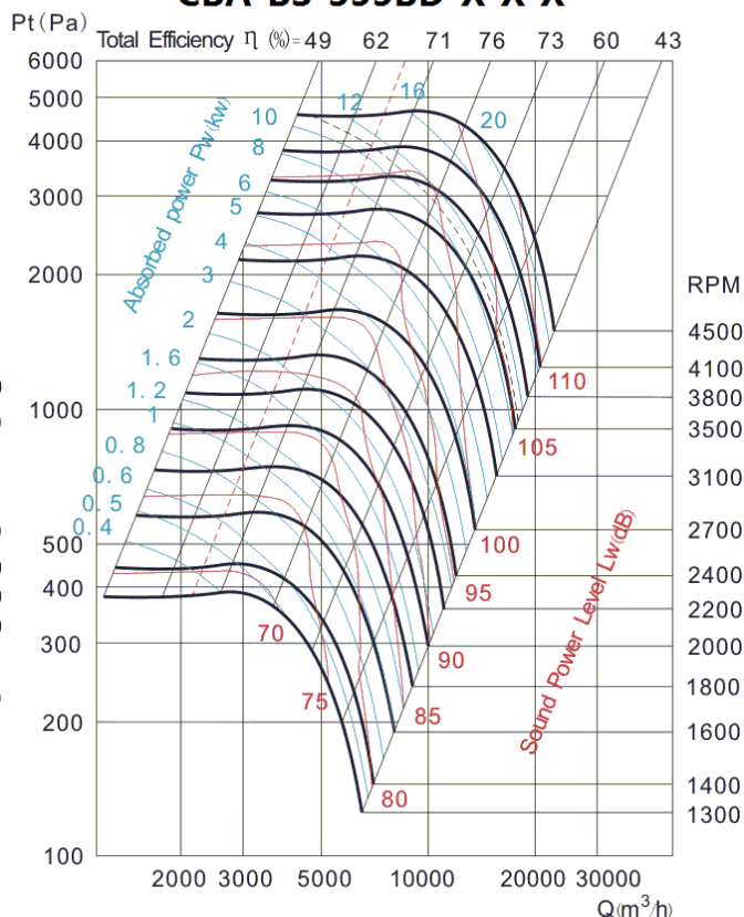
CBA-BS-355BD-X-X-X
