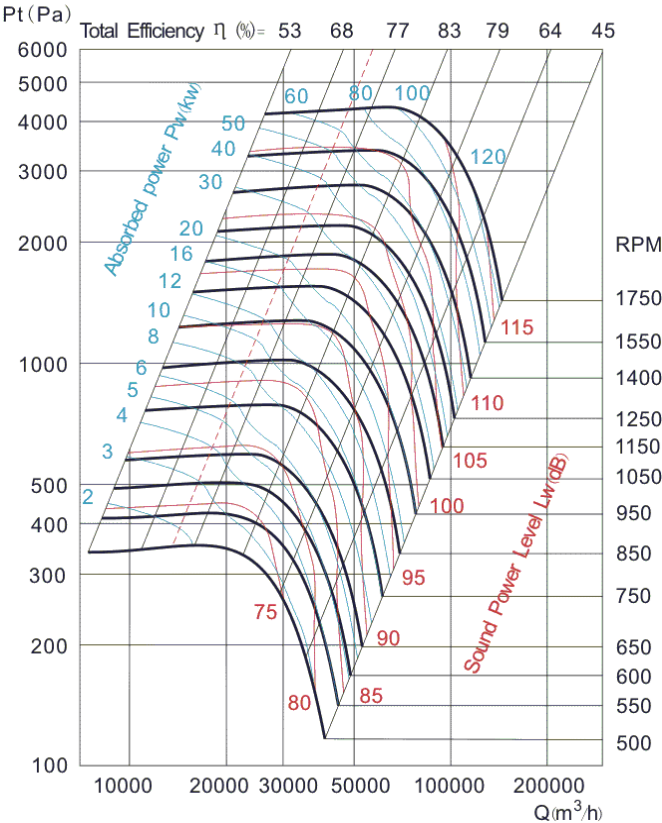
CBA-BS-900BD-X-X-X
