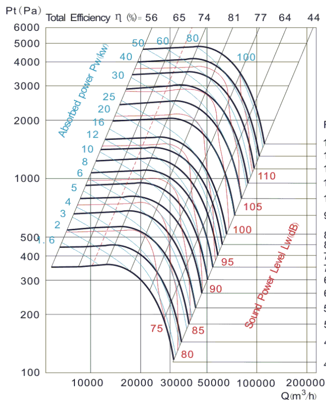
CBA-BA-1400BS-X-X-X
