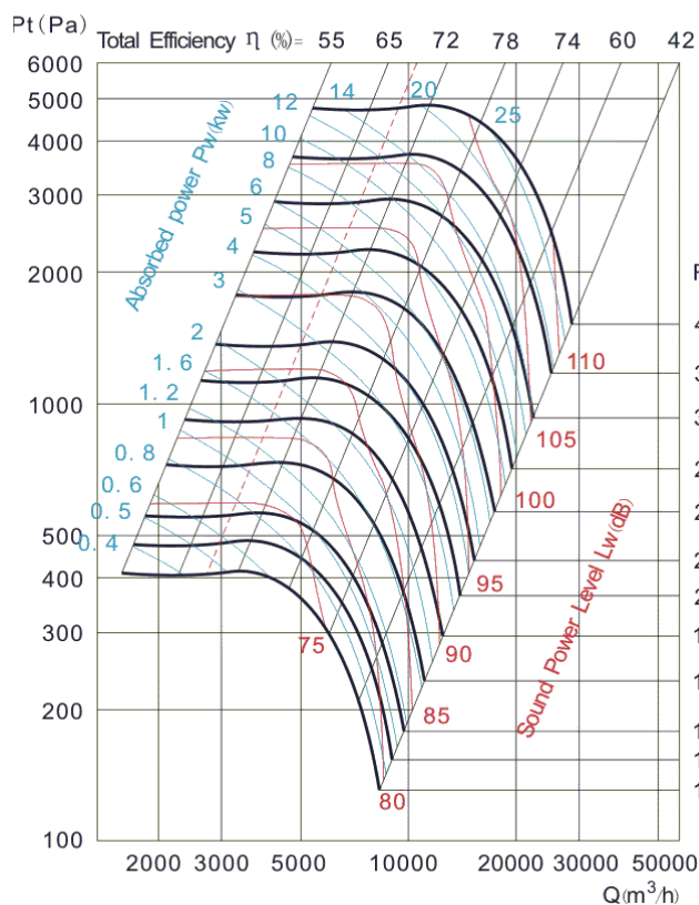
CBA-BS-400BD-X-X-X
